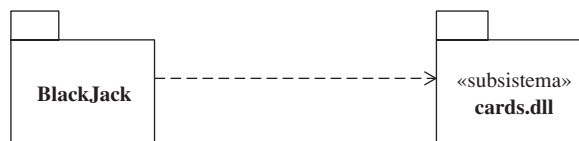
Figura 5-14 El diagrama muestra que el paquete “BlackJack” depende del paquete “cards.dll”, en el cual se usa el estereotipo «subsistema».
