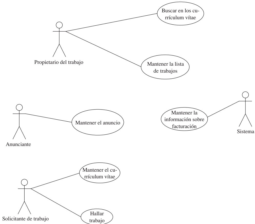
Figura 2-12 Esta figura sugiere que los trabajos, los currículum vitae y los anuncios son todos listas que debe mantener un propietario de lista, así como una asociación entre el sistema de facturación y las listas y las búsquedas de los currículum vitae.
