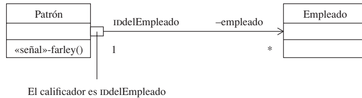
Figura 6-15 El calificador que da como resultado un empleado único es el “IDdelEmpleado”.
