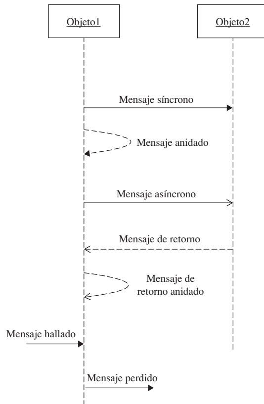
Figura 4-3 Símbolos de llamadas de los métodos síncrono y asíncrono.
